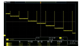
ISO16750电压骤降复位特性
