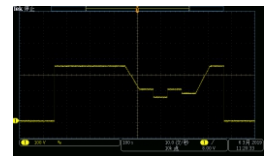
VW80300 EHV-03欠电压操作
