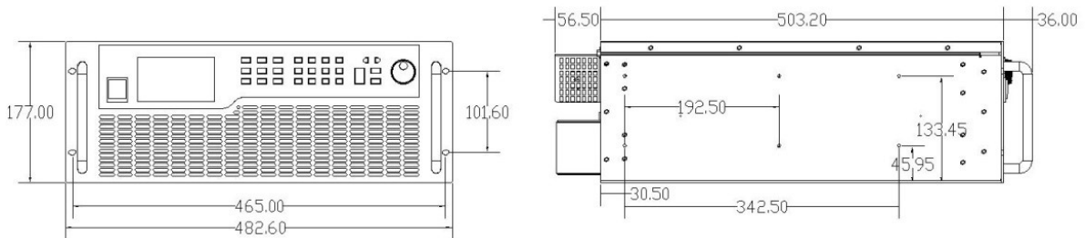
6. 5kW机型尺寸图（40V~1500V机型）：
