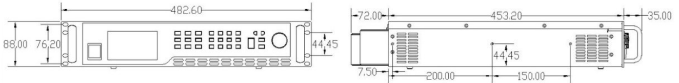
2kW、3.2kW机型尺寸图（40V~1500V机型）：
