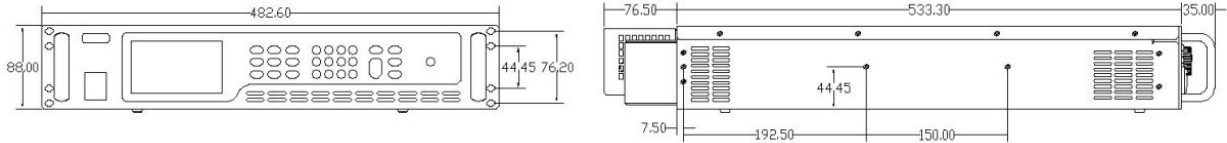
2kW、3.2kW机型尺寸图（40V~1500V机型）：
