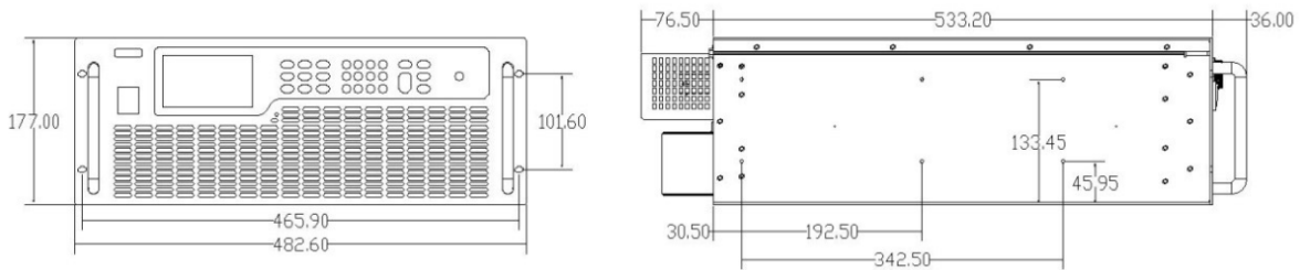
4. 8kW、6.5kW机型尺寸图（10V~30V机型）：
